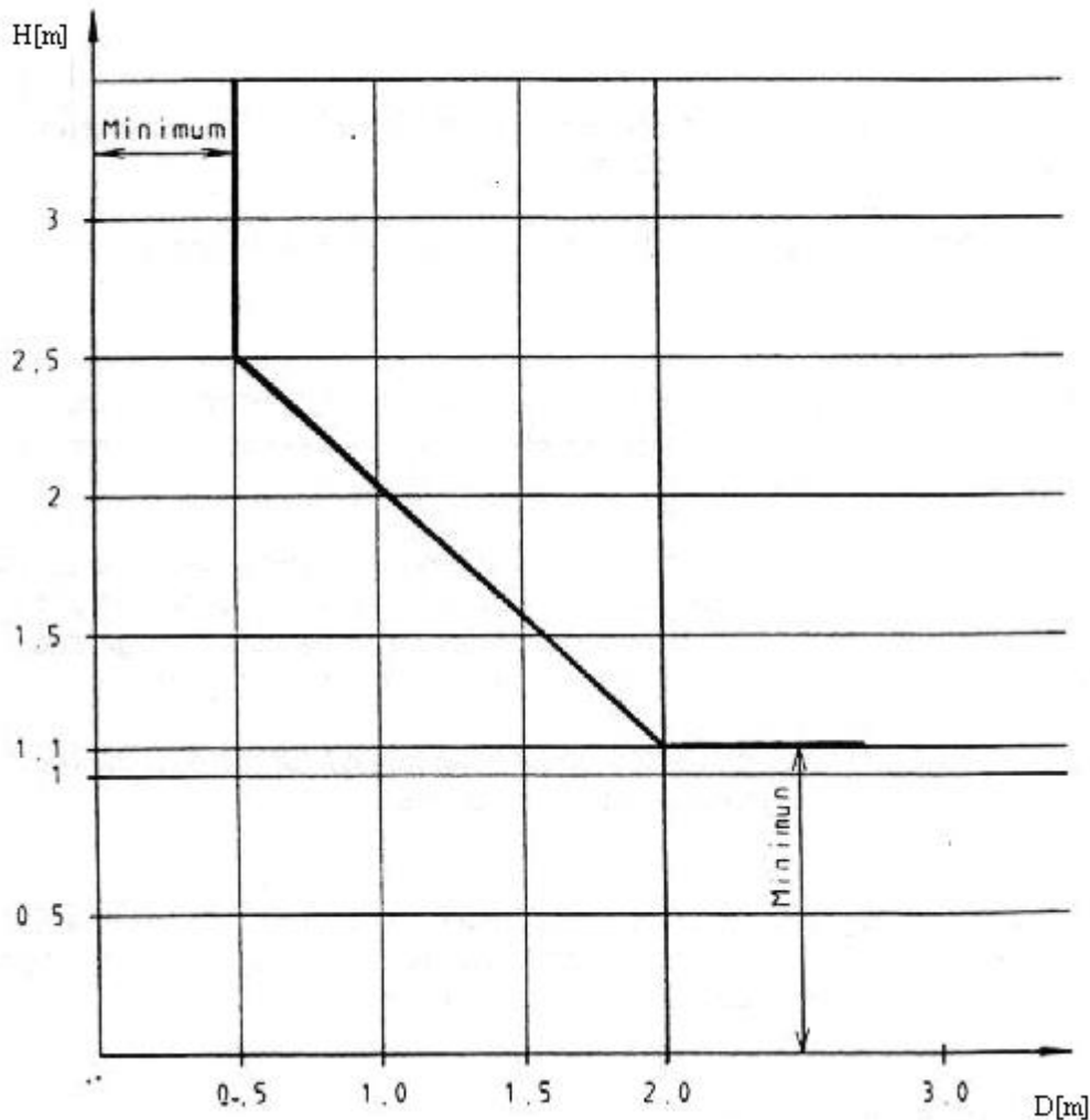
شکل 2: چاه نیمه پوشیده - فواصل
